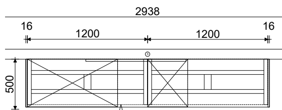
Draufsicht / Bovenaanzicht / Vue du dessus / Plan view
