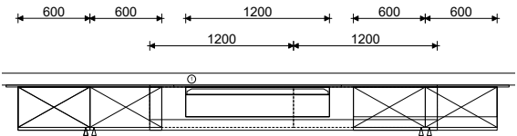
Draufsicht / Bovenaanzicht / Vue du dessus / Plan view
