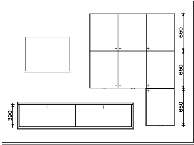
Frontansicht / Frontaanzicht / Vue de face / Front view
