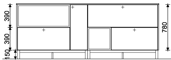
Frontansicht / Frontaanzicht / Vue de face / Front view
