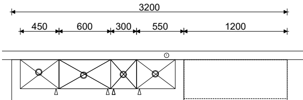
Draufsicht / Bovenaanzicht / Vue du dessus / Plan view
